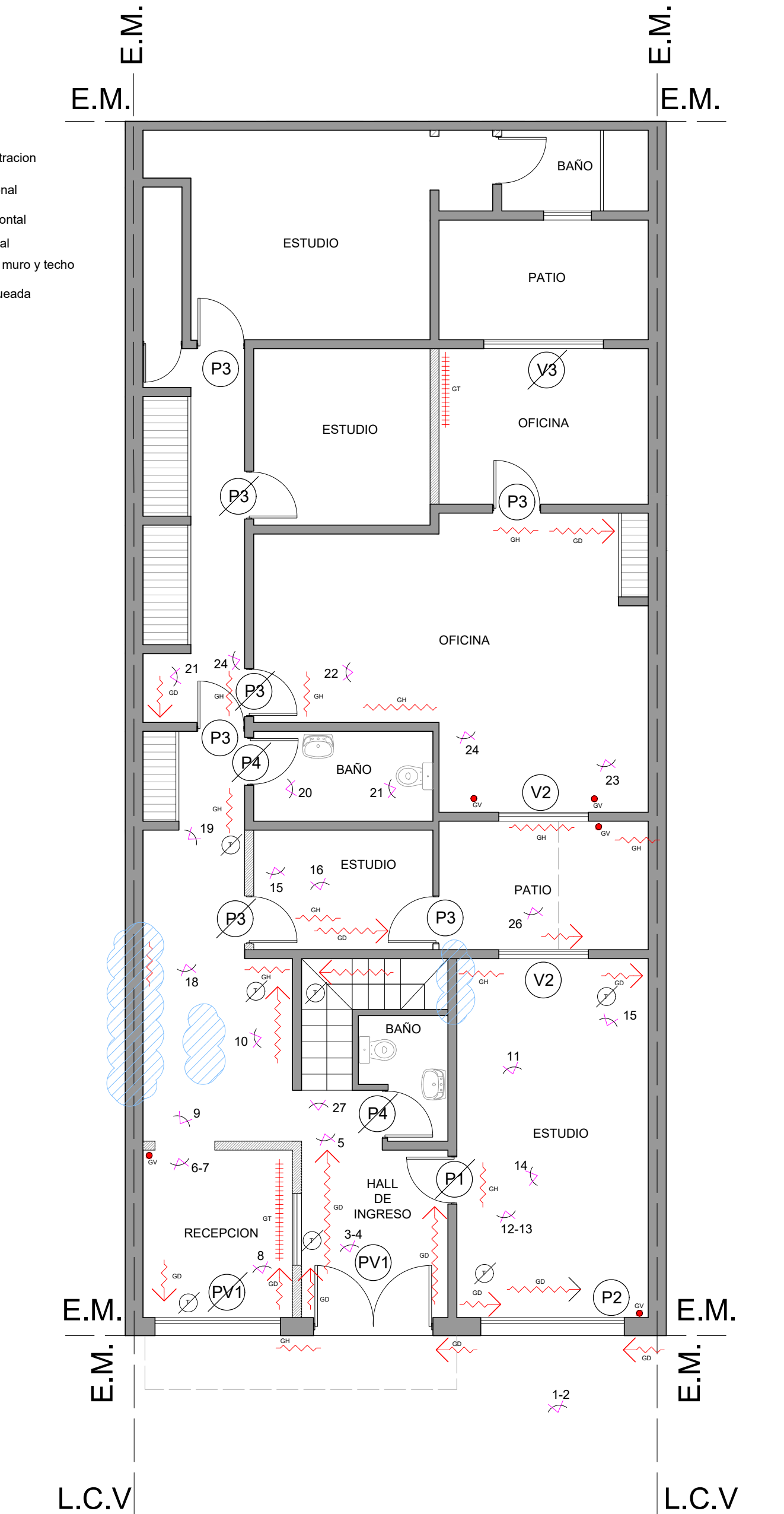
PLANTA BAJA
