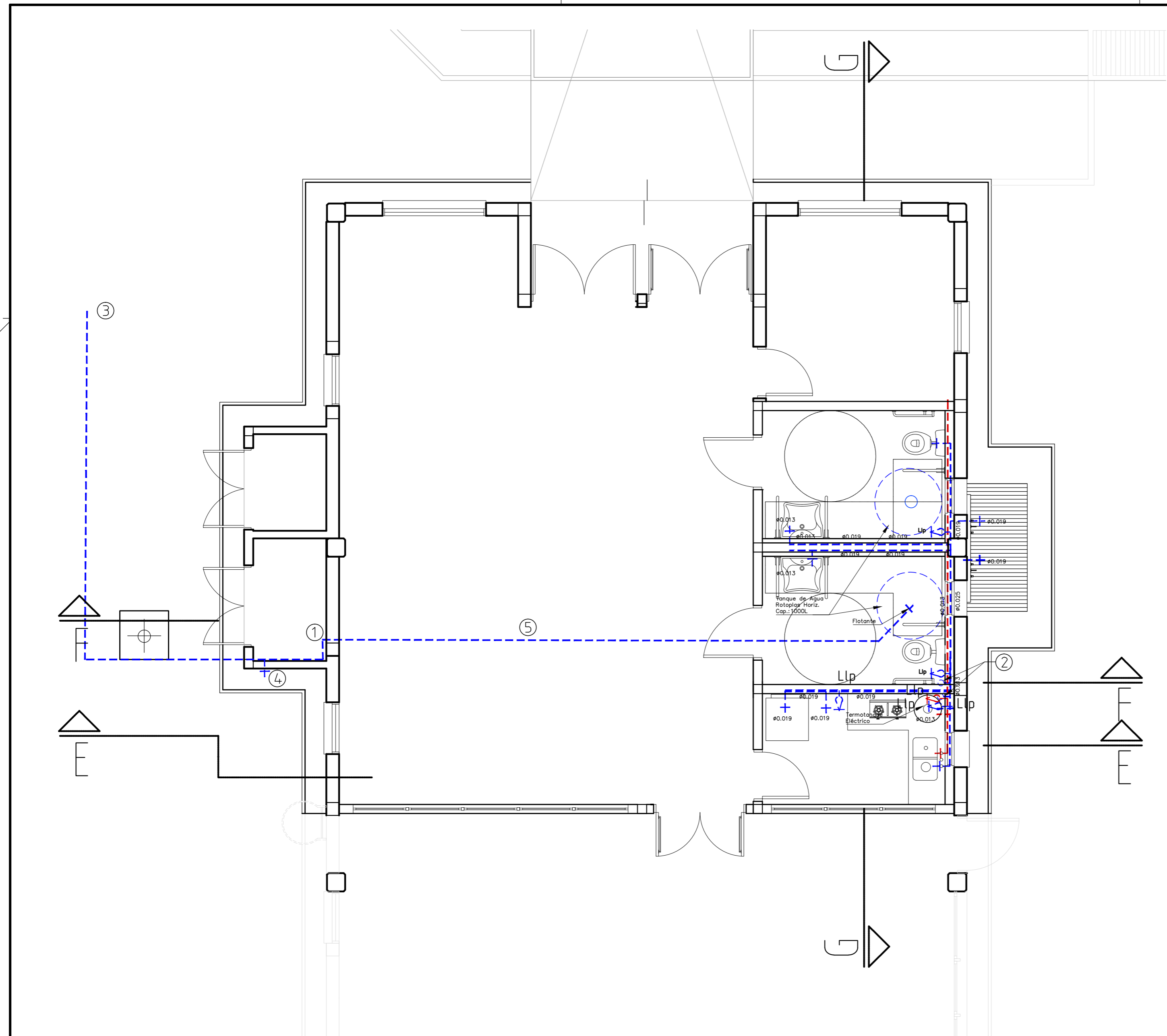
PLANTA INSTALACIÓN DE AGUA
