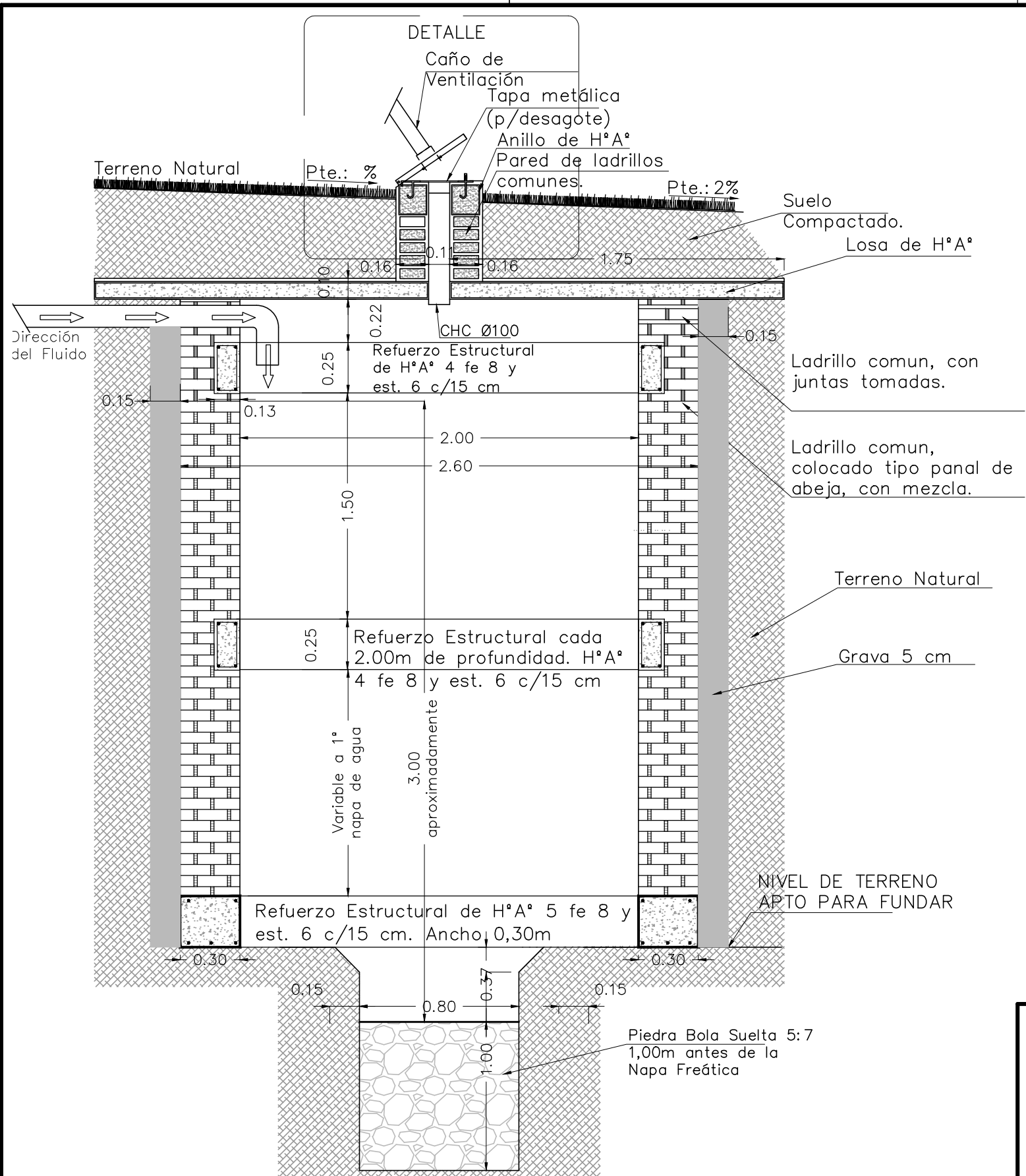
POZO ABSORBENTE (corte transversal)
