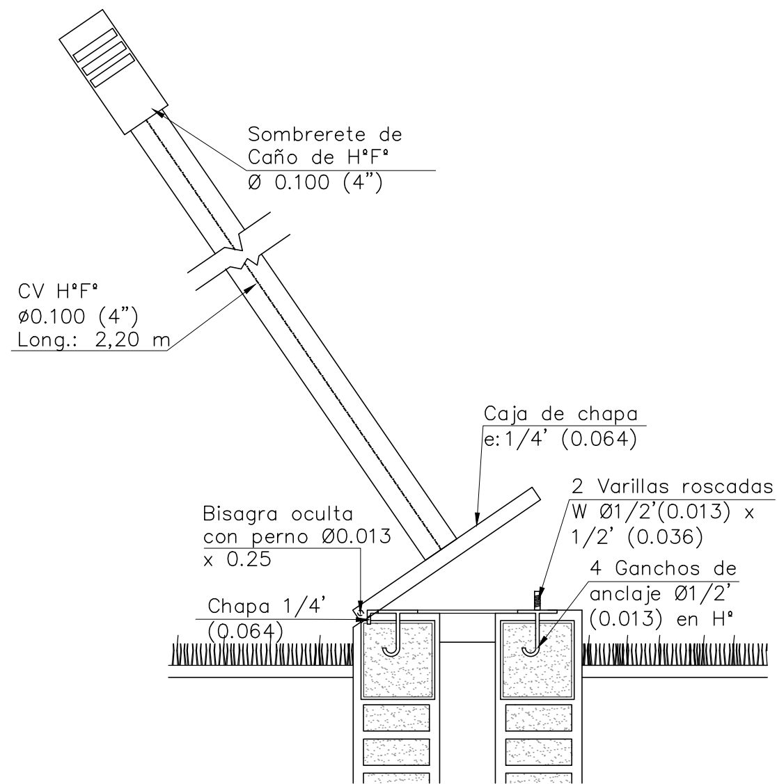
DETALLE DE P.A.C. Esc.: 1:10
