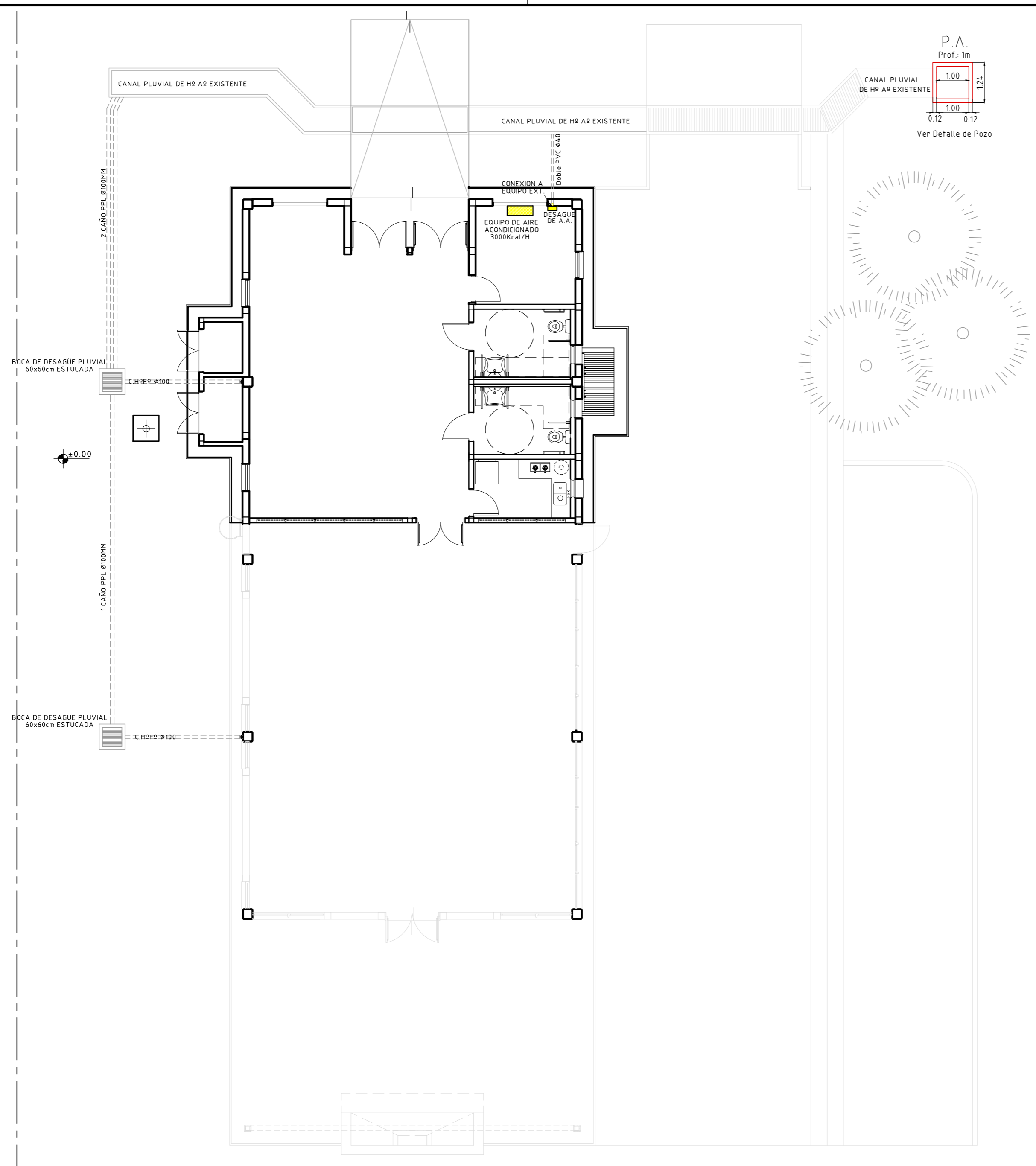
PLANTA INST. ELECTRICA - EQUIPOS DE AIRE ACOND. Y DESAGÜES
